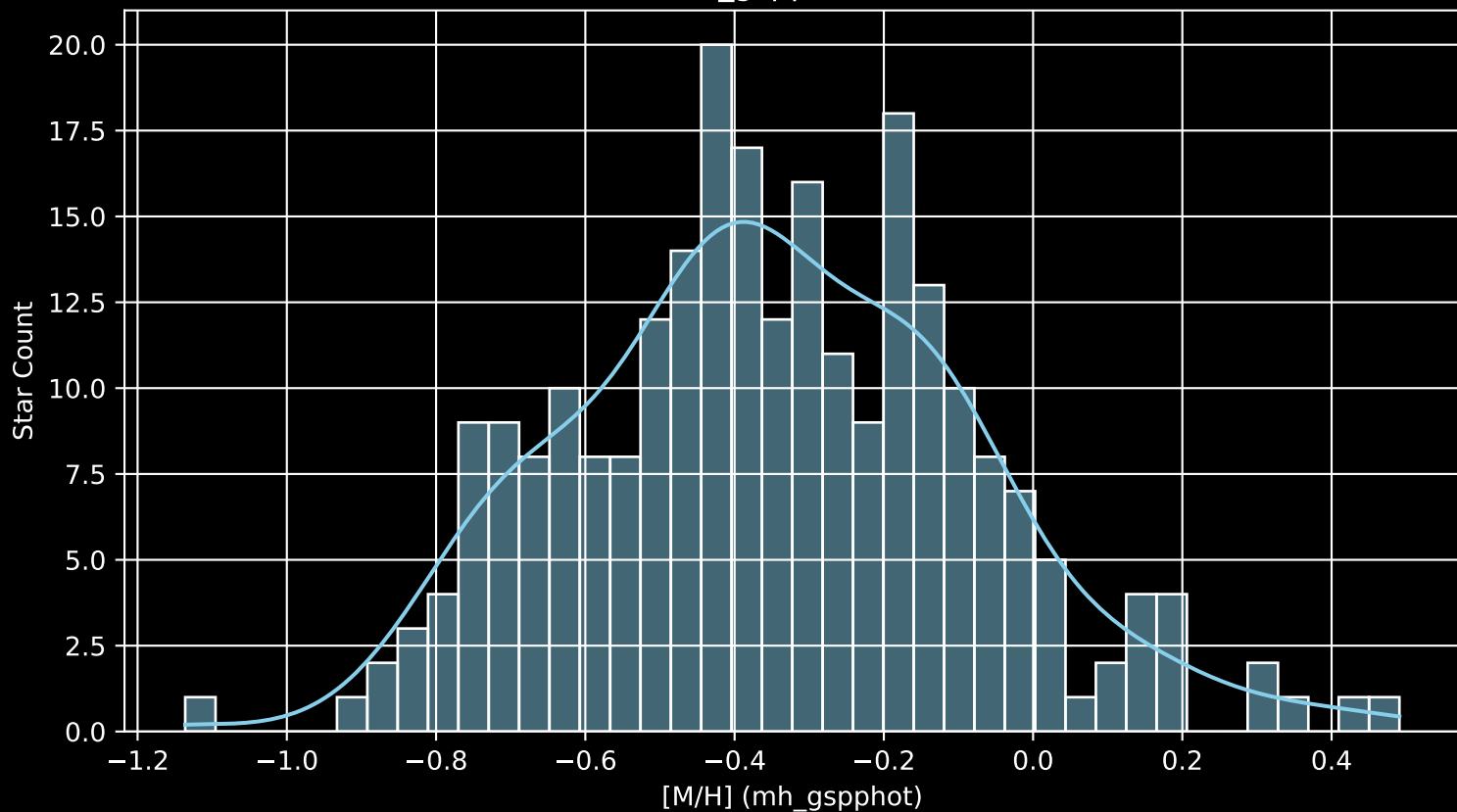
GALAH DR4 Field: [3237] [M/H] (mh_gspphot) (n= 251)
