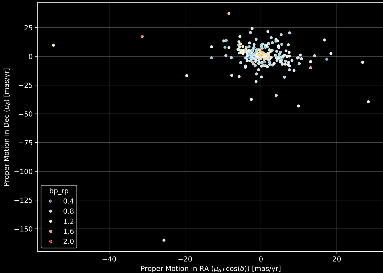
GALAH DR4 Field: [3237] Proper Motion Diagram (n= 252)
