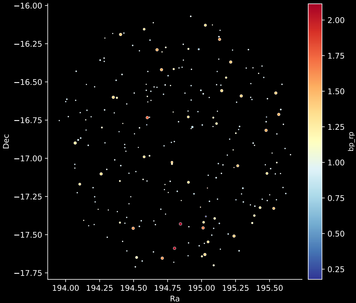
GALAH DR4 Field: [3237] Stars: 252
