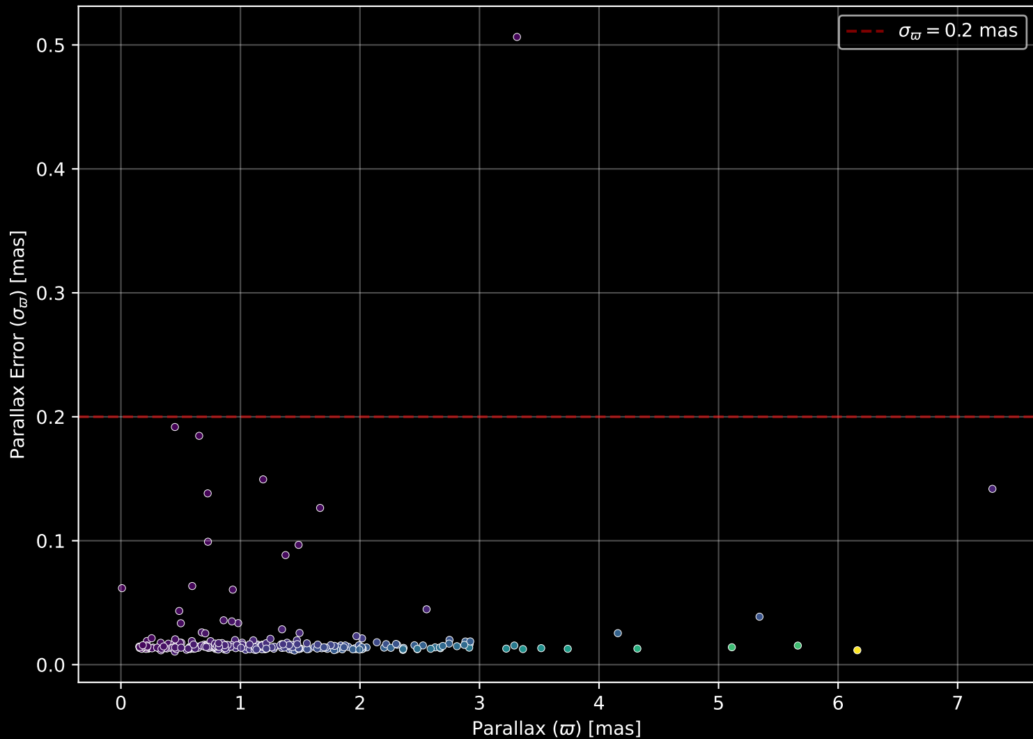
GALAH DR4 Field: [3237] Parallax Quality (n= 252)
